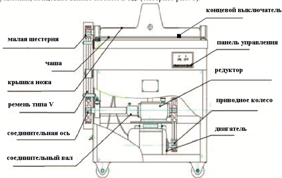
Рис. 1 Основные механизмы оборудования
